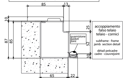
TELAIO PIATTO CON COPRIFILI - ESTRUSIONE 10 mm DAL MURO INTERNO FLAT FRAME WITH EDGING TRIMS - EXTRUSION 10 mm FROM THE INTERNAL WALL CADRE PLAT AVEC COUVRE-JOINT - EXTRUSION 10 mm SUR MUR INTERIEUR
