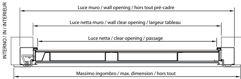
SEZIONE ORIZZONTALE HORIZONTAL SECTION COUPE HORIZONTALE
